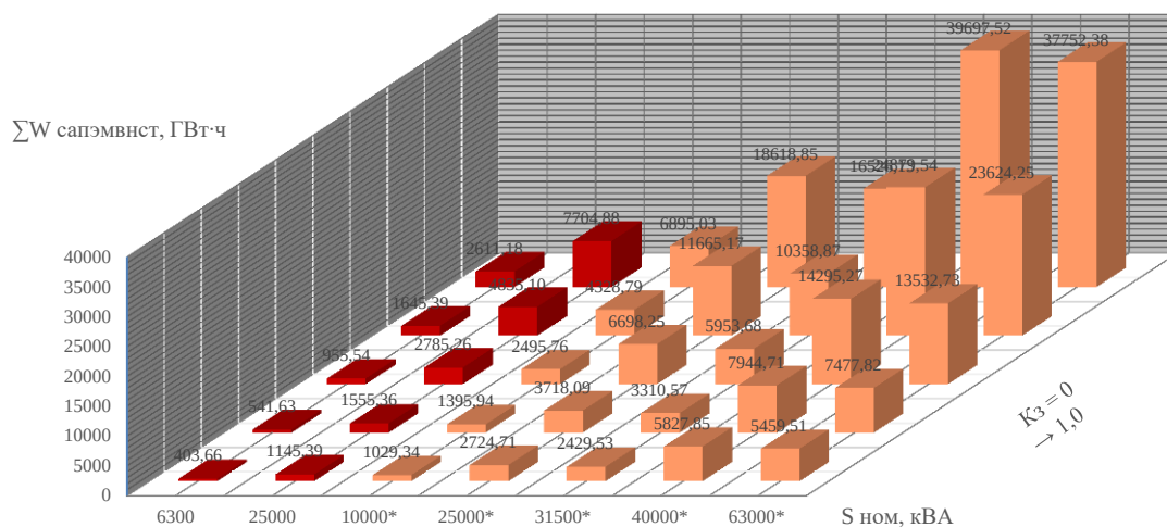
Рис. 5. Диаграмма аллокации САПЭМВН от полной мощности модифицированного сортамента, сгруппированного из серий S(F)Z13 и SS(F)Z13, интегрируемых в ПП Краснолучского ОЭС – 110 кВ, определенных при колебаниях спокойной нагрузки в исследуемых границах \Sigma W_{\text{САПЭМВН.СТ}} = f(S_{\text{ном}})
