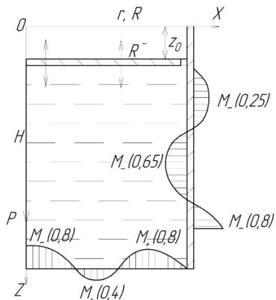
Рис. 3. Эпюра изгибающего момента M_- вдоль сопряжения вертикальных несущих панелей емкости с плавающей крышей натурального объекта [6]
