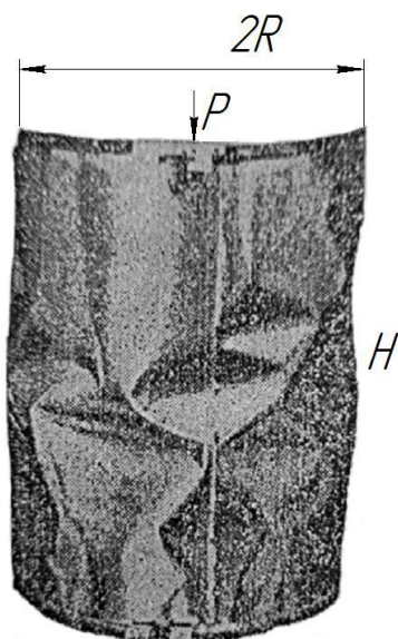
Рис. 4. Максимальная интенсивность выпучивания резервуара в нижней его части [6] с последующим волнообразованием
