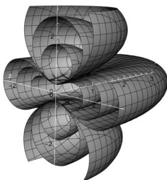
Рис. 11. Пространственная конфигурация поля квадрупольного
