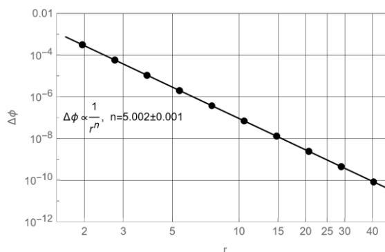
Рис. 12. Зависимость величины ошибки от расстояния для квадрупольного
