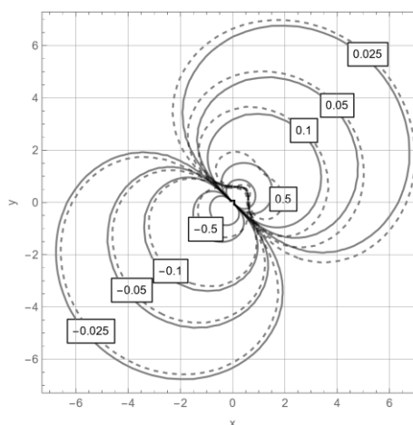
Рис. 6. Эквипотенциальные линии диполя
