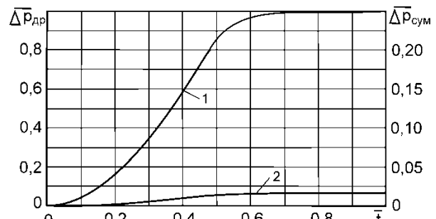
Рис. 4. Результаты расчёта составляющих давления p_2 :
