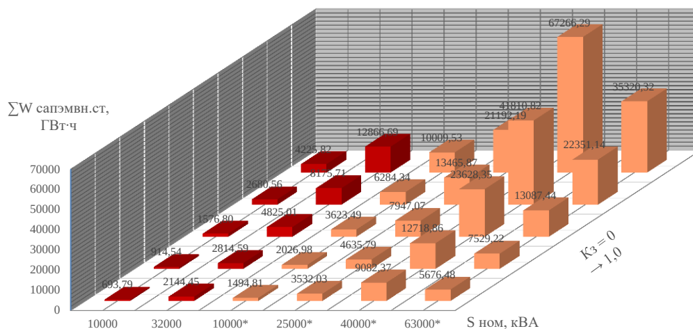
Рис. 14. Диаграмма аллокации САПЭМВН от полной мощности модифицированного сортамента, сгруппированного из серий ТДН и ТДТН, интегрируемых в ПП Краснолучского ОЭС – 110 кВ, определенных при колебаниях спокойной нагрузки в исследуемых границах \Sigma W_{САПЭМВН.СТ} = f(S_{ном})
