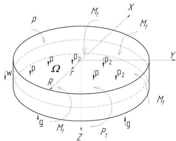
Рис. 1. Опорная частично заглубленная плита весом P_1 с емкостью, заполненной жидкостью весом P_2 = \rho(H - z_0) , где \rho – плотность жидкости; z_0 – высота резервуара, незаполненная жидкостью
