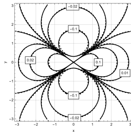
Рис. 10. Эквипотенциальные линии квадруполь
