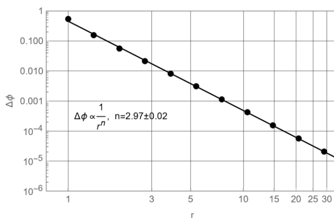
Рис. 4. Зависимость величины ошибки от расстояния для монополя
