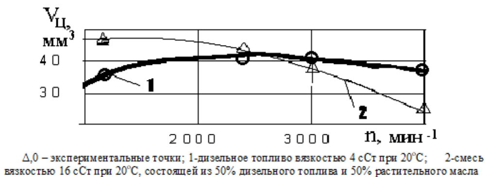
Рис. 1. Экспериментальные скоростные характеристики топливоподачи
