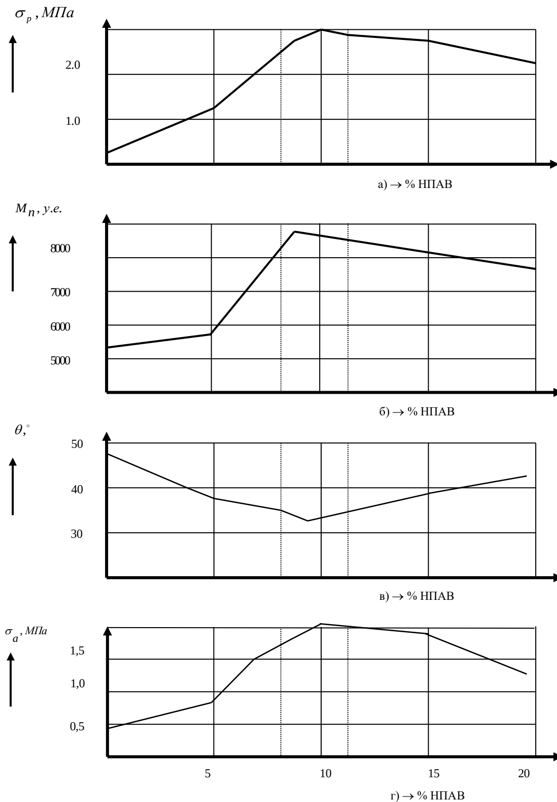
Рис.3. Показатели влияния модификатора из класса НПАВ на свойства ЛСТ: а – на связующую способность, б – на изменение молекулярной массы, в – на изменение краевого угла смачивания, г – на изменение сил адгезии
