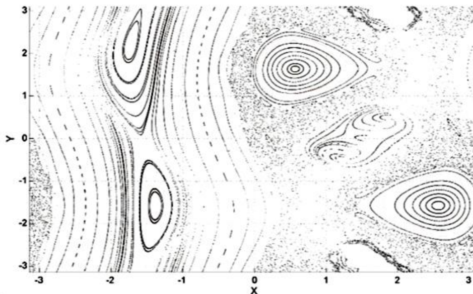
Рис. 2. Сечение Пуанкаре линий тока ABC-течения при z=0
