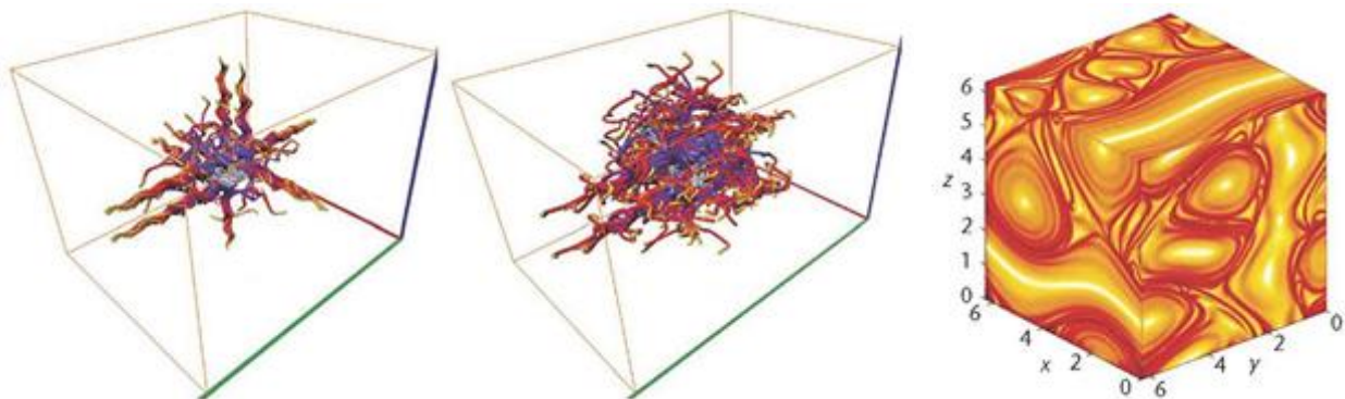
Рис. 1. Визуализация путей линий АВС-течения в последовательные интервалы времени и в проекции на координатные плоскости
