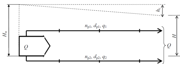
Рис. 3. Расчетная схема рукавной системы с параллельной прокладкой рукавных линий
