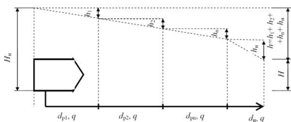
Рис. 2. Расчетная схема рукавной системы с последовательным соединением рукавов
