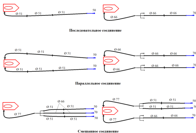
Рис. 1. Основные схемы насосно-рукавных систем
