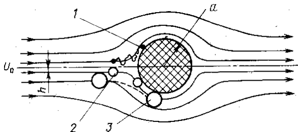
Рис. 1. Схема механизмов осаждения аэрозольных частиц из газовоздушного потока, обтекающего одиночный фильтр:
