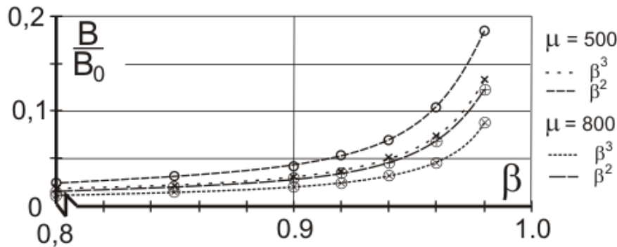
Рис. 3. Зависимости эффективности экранирования от соотношения внутреннего радиуса экрана к внешнему для стальных экранов с \mu = 500 и 800
