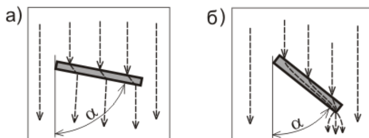
Рис. 2. Картины магнитного поля при наличии наклонённой плоской ферромагнитной пластины
