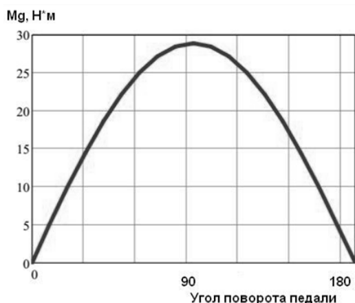
Рис. 2. Изменение крутящего момента за пол-оборота одной педали на ведущей звездочке
