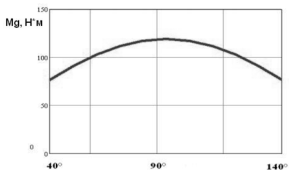
Рис. 5. Изменение величины крутящего момента в зависимости от перемещения педали маятникового привода
