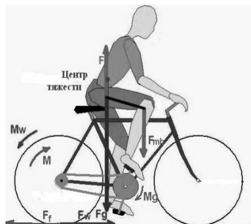
Рис. 1. Силы и моменты сил при движении системы «велосипед+велосипедист»
