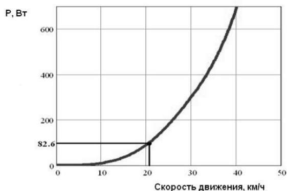
Рис. 3. Графическое определение скорости движения велосипедиста с традиционным pedalным приводом
