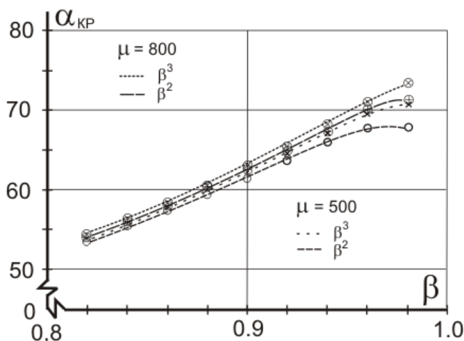
Рис. 5. Зависимости значений \alpha_{кр} от \beta при относительной магнитной проницаемости экрана, равной 500 и 800
