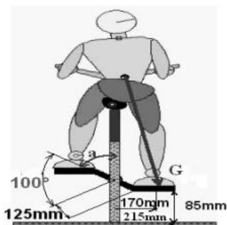
Рис. 4. Основные расчетные параметры маятникового pedalного привода
