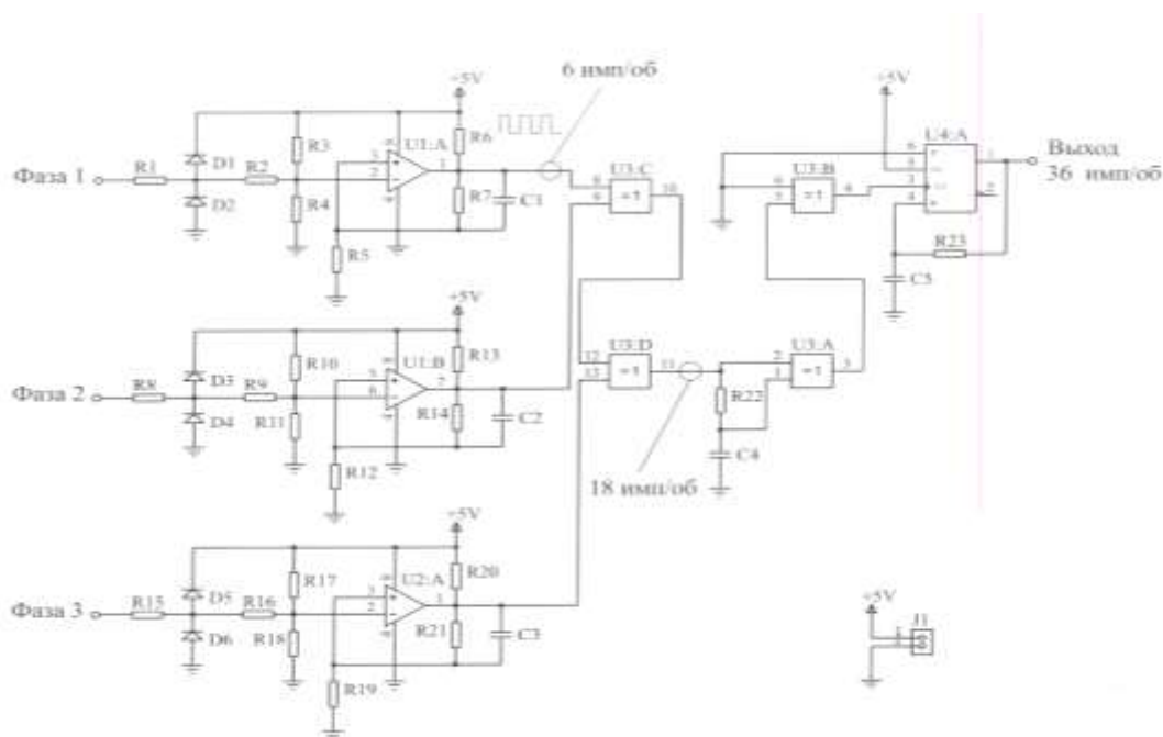
Рис. 1. Схема формирователя импульсов
