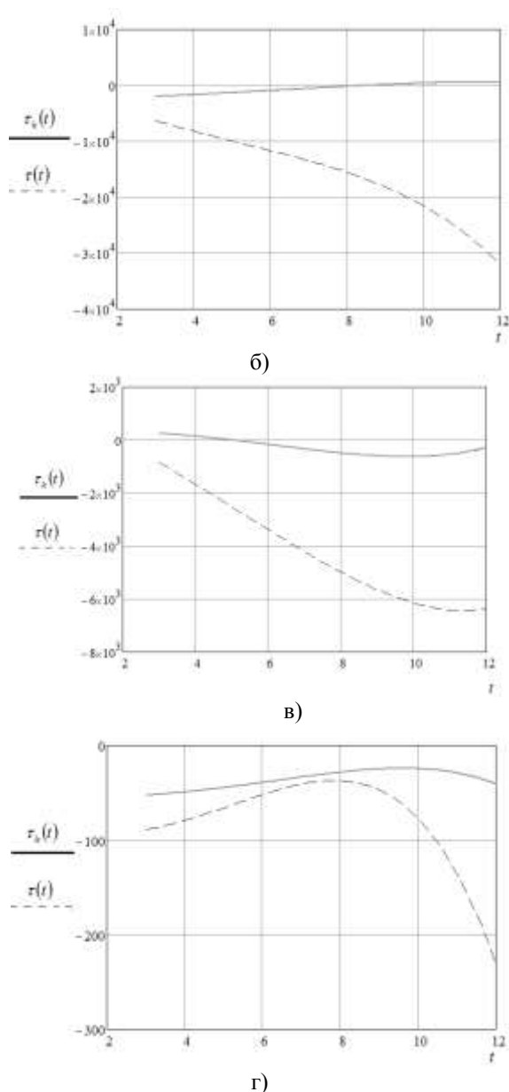
Рис. 3. Изменения величины фактического \tau(t) и скорректированного \tau_k(t) моментов для: а) первой степени подвижности; б) второй степени подвижности; в) третьей степени подвижности; г) четвертой степени подвижности
