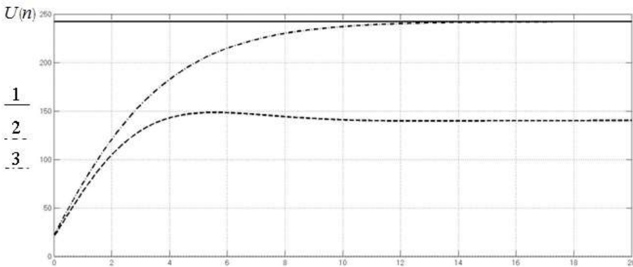
Рис. 5. Управляющее воздействие в системе автоматического управления температурой в процессе гомогенизации молока:
