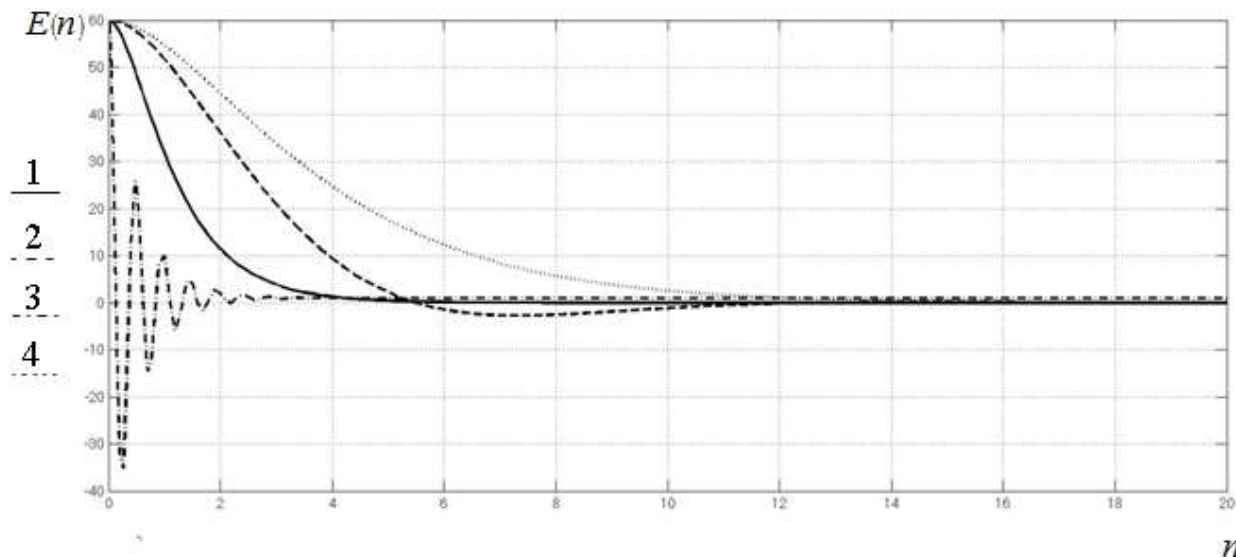
Рис. 7. Величина рассогласования в системе автоматического управления температурой в процессе гомогенизации молока:
