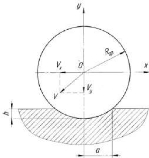
Рис. 1. Упругое внедрение гранулы в обрабатываемую поверхность
