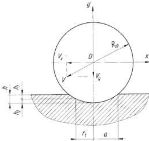
Рис. 2. Упругопластическое внедрение гранулы в обрабатываемую поверхность при выполнении условия:
