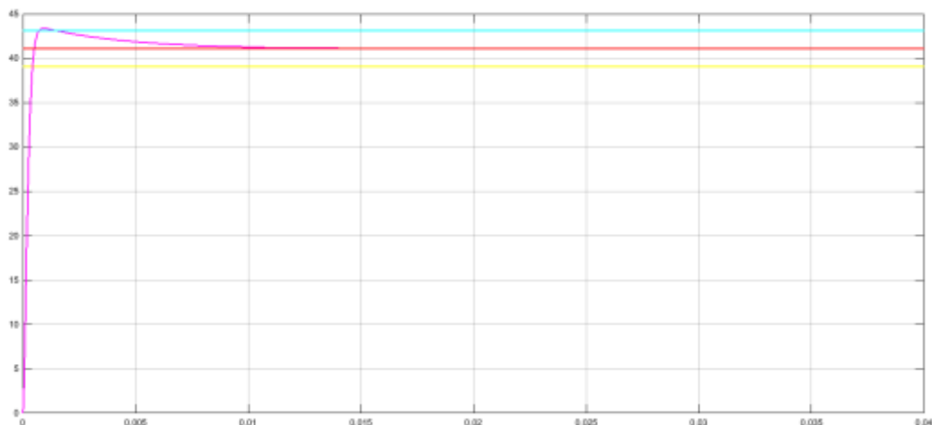
Рис. 5. Переходная характеристика САУ двигателем постоянного тока для второй степени подвижности манипулятора с цилиндрической БСК
