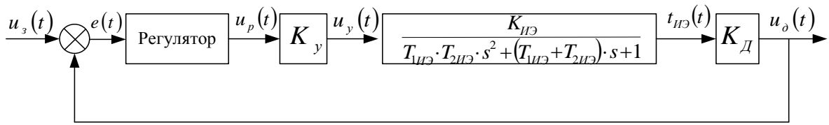
Рис. 2. Структурная схема системы автоматического управления технологическим процессом нагрева молока
