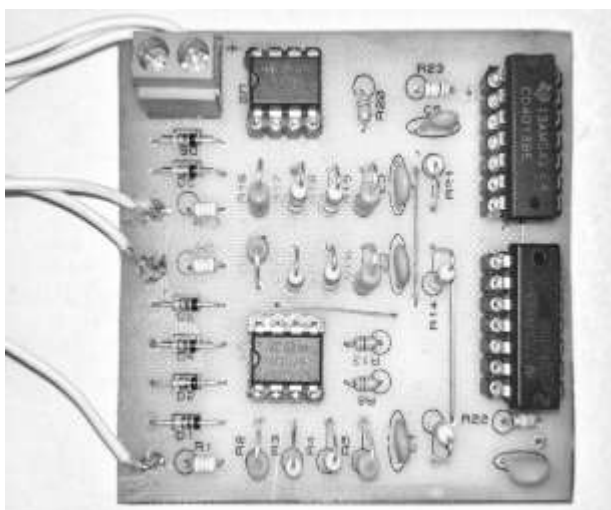
Рис. 3. Печатная плата формирователя счётных импульсов
