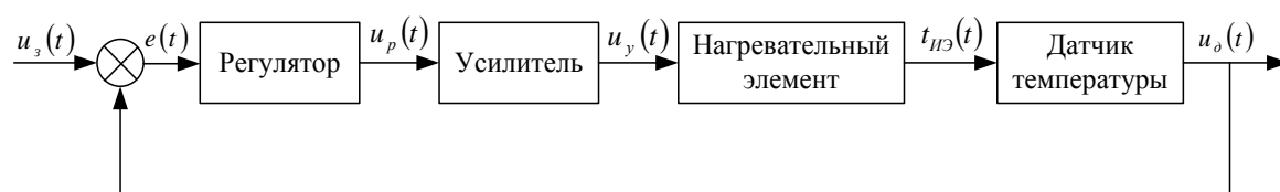
Рис. 1. Функциональная схема системы автоматического управления технологическим процессом нагрева молока
