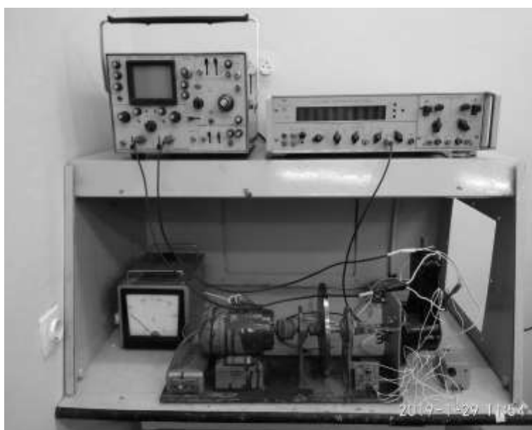
Рис. 2. Стенд для испытаний тахогенераторов
