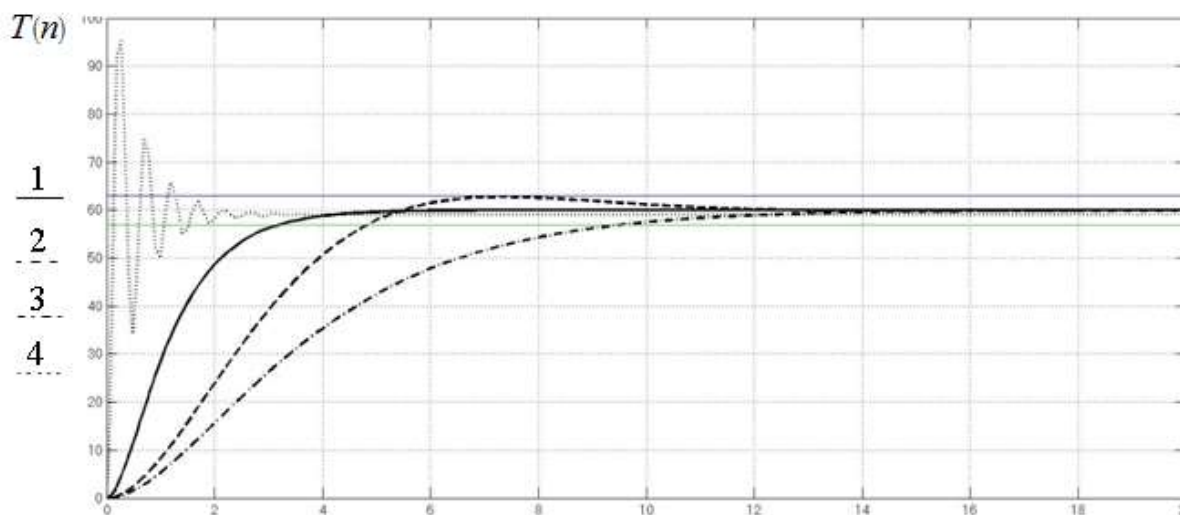
Рис. 6. Переходной процесс в системе автоматического управления температурой в процессе гомогенизации молока:
