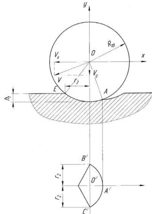
Рис. 3. Упругопластическое внедрение гранулы в обрабатываемую поверхность при нарушении условия:
