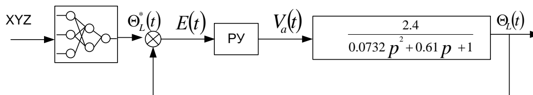
Рис. 2. Структурная схема системы управления двигателем постоянного тока звена манипулятора
