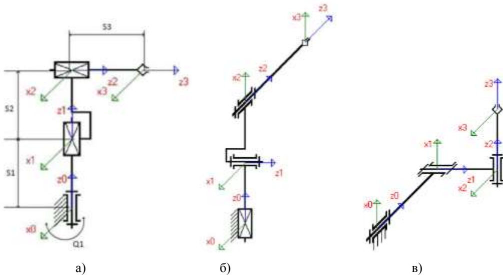
Рис.1. Структурные схема манипуляторов а) цилиндрическая БСК; б) сферическая БСК; в) ангулярная БСК
