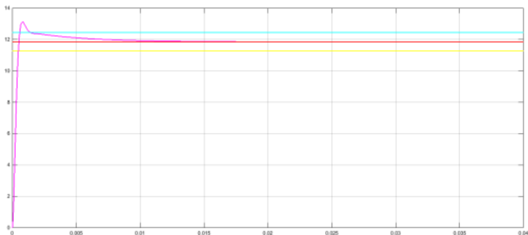
Рис. 4. Переходная характеристика САУ двигателем постоянного тока для первой степени подвижности манипулятора с цилиндрической БСК
