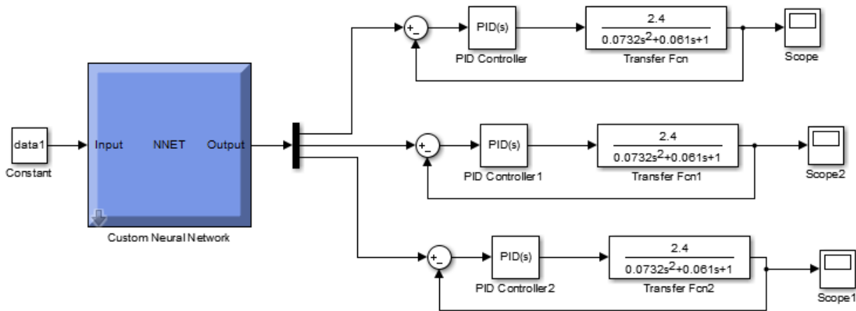
Рис. 3. Simulink-модель системы управления двигателями звеньев манипулятора
