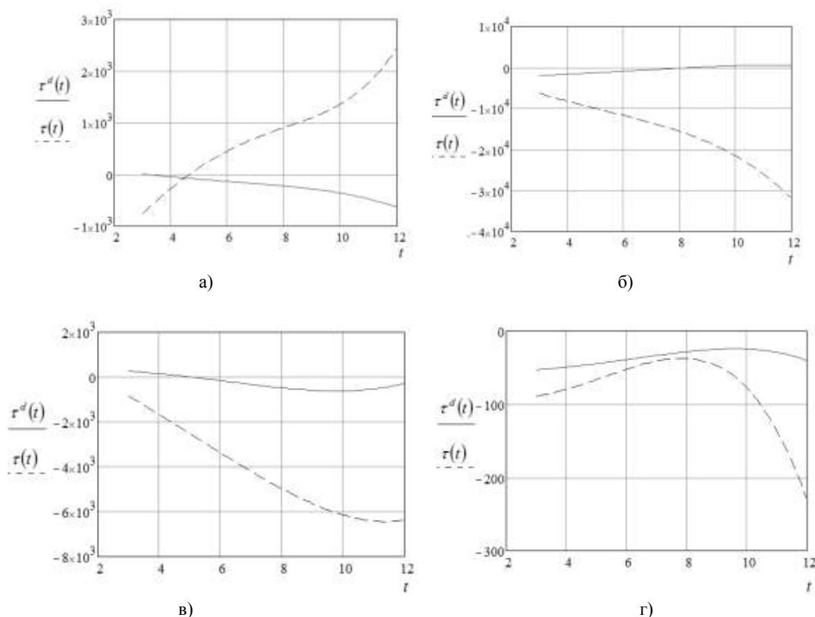
Рис. 2. Изменения величины требуемого \tau^d(t) и фактического \tau(t) моментов для: а) первой степени подвижности; б) второй степени подвижности; в) третьей степени подвижности; г) четвертой степени подвижности
