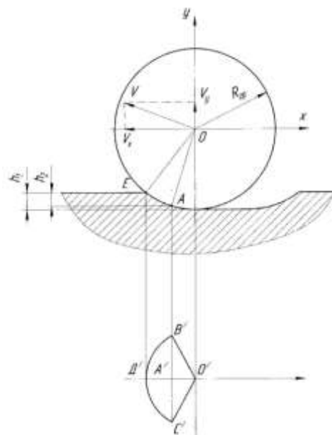
Рис. 4. Упругопластический или упругий выход гранулы из контакта
