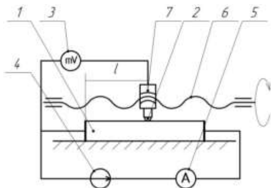
Рис. 1. Схема измерения удельного электросопротивления вдоль длины градиентного кристалла сплава Sb-Bi:
