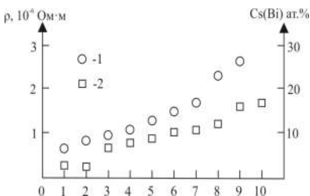
Рис. 2. Зависимость удельного электросопротивления и концентрации висмута в твёрдой фазе от длины кристалла: 1 - удельное электросопротивление; 2 - концентрация висмута в твёрдой фазе
