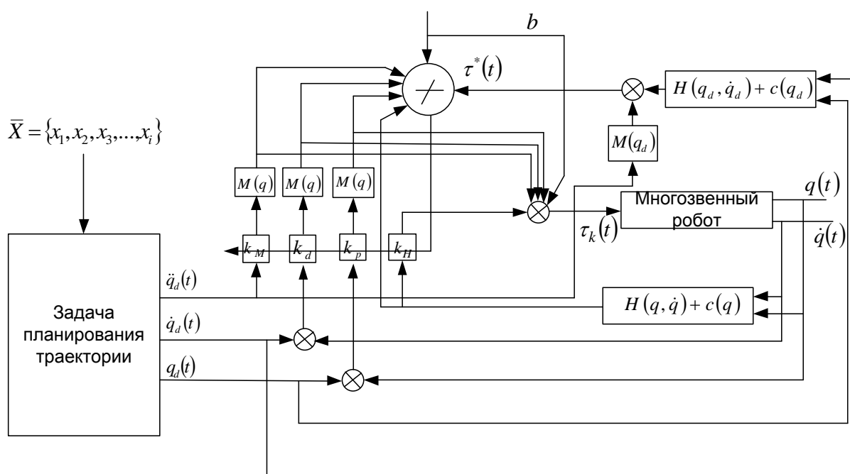
Рис. 1. Структурная схема системы управления по методу вычисляемого момента с нейронным способом настройки коэффициентов
