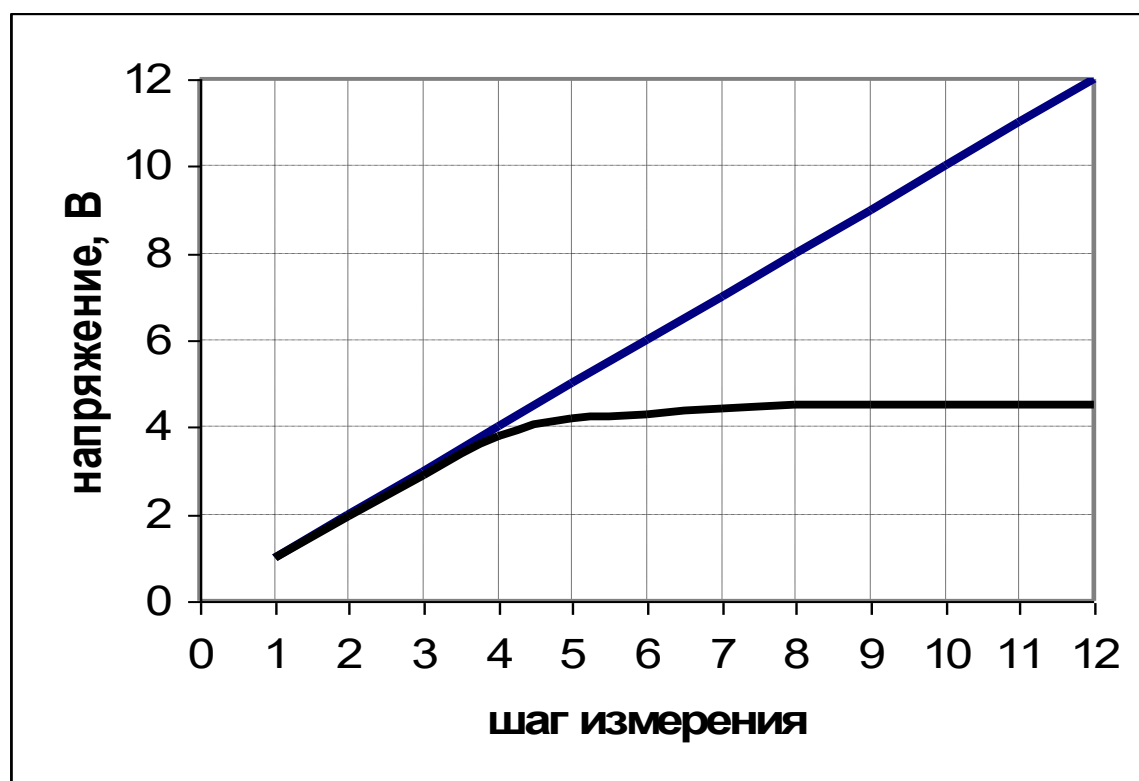
Рис. 6. Рабочая характеристика схемы
