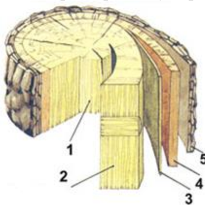
Рисунок 1 – Строение древесины
